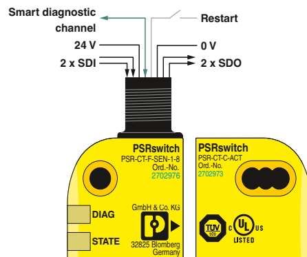
Интеллектуальный датчик
