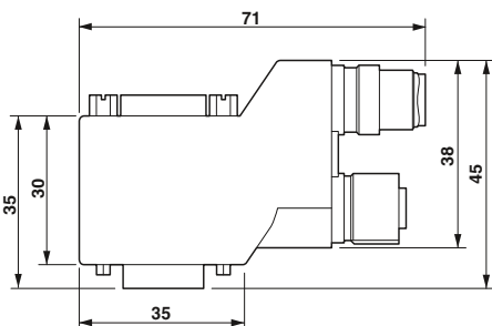
Размерный чертеж SUBCON-PLUS...90...M12, короткий модель 90°
