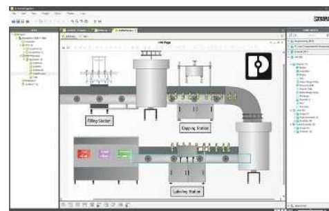
Визуализация
